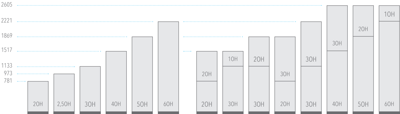
Schränke auf Stahlsockel, 45 mm hoch
